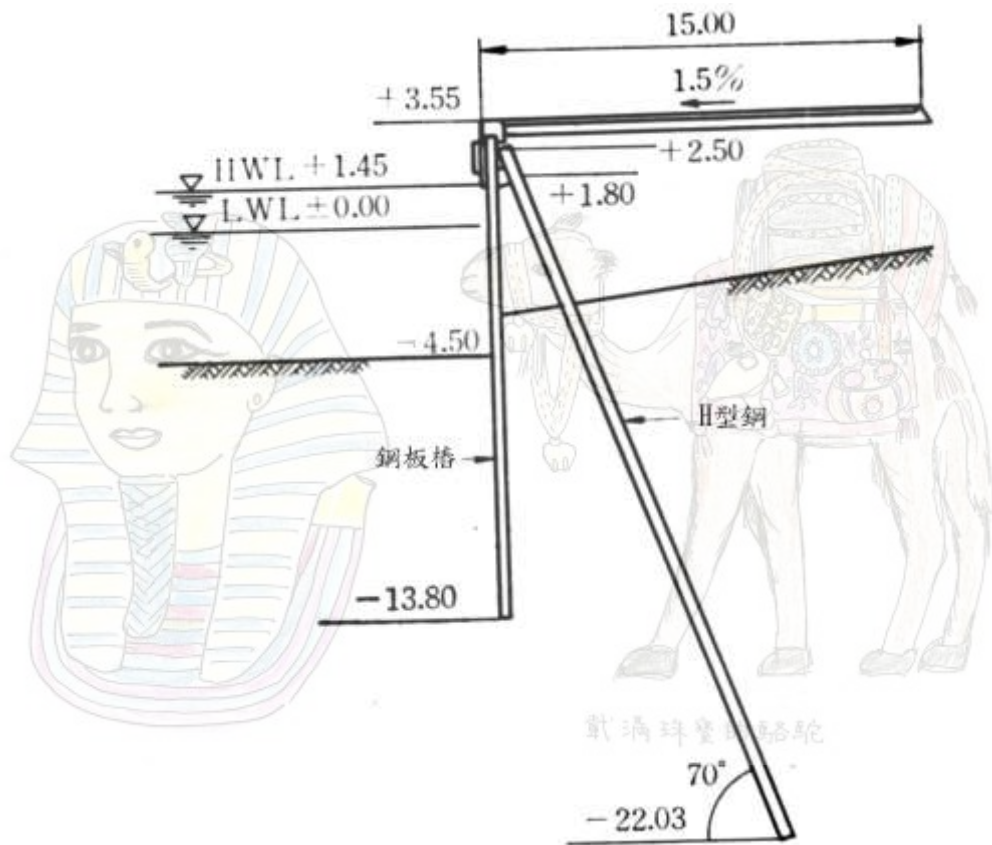
2011 斜錨樁板樁式碼頭
